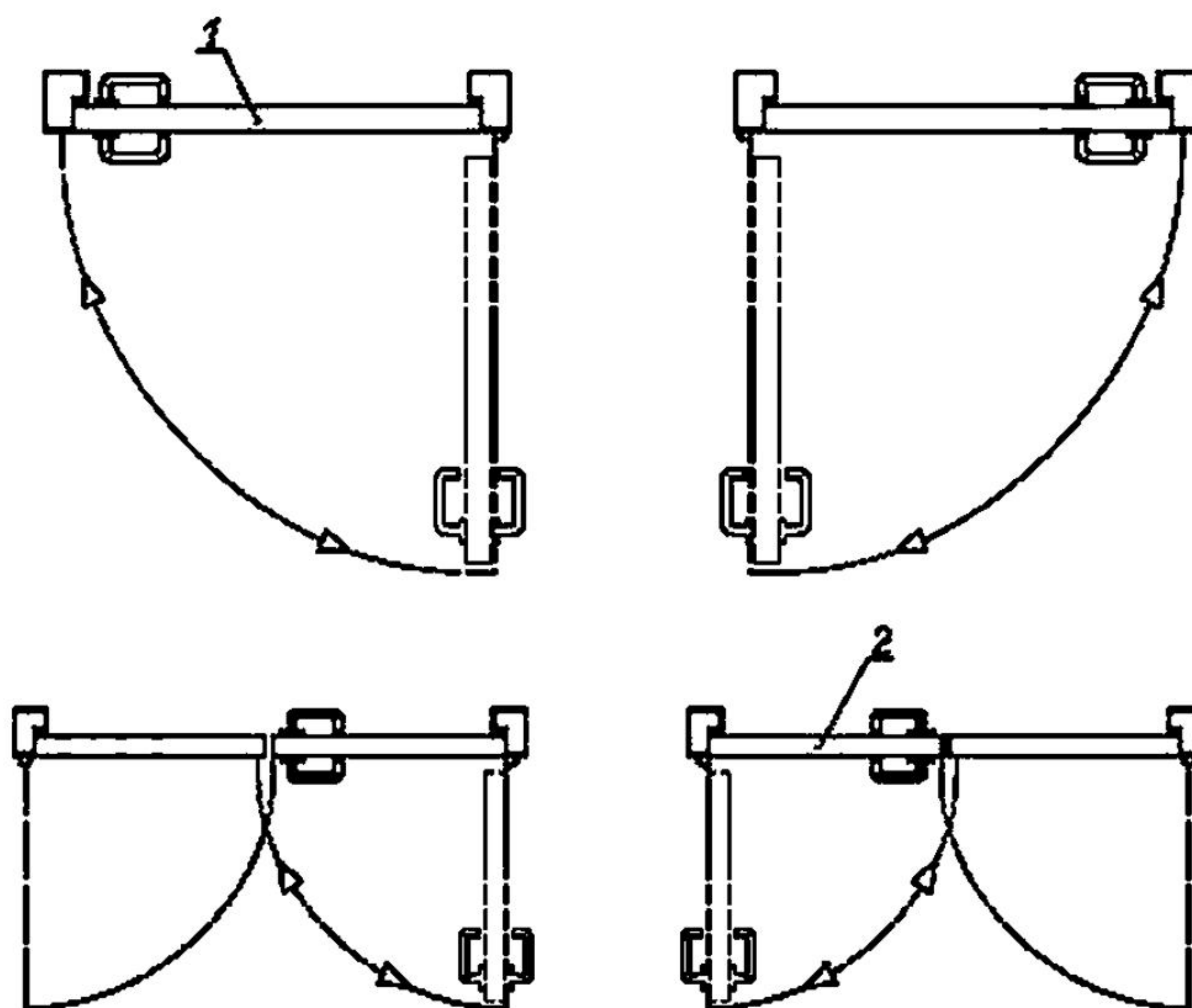
Рисунок А.3 — Примеры направления открывания дверей
