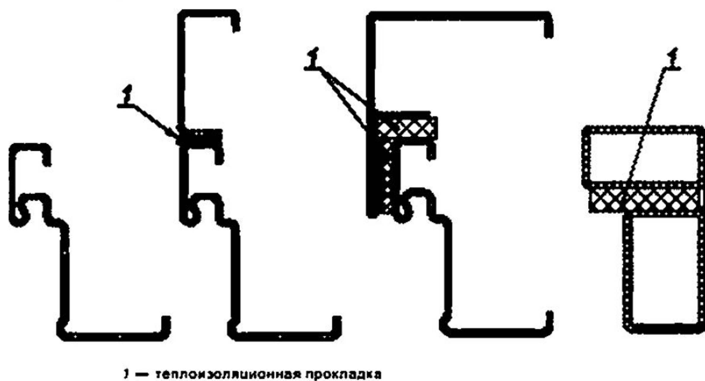
Рисунок Б.1 — Примеры конструктивного исполнения дверных коробок
