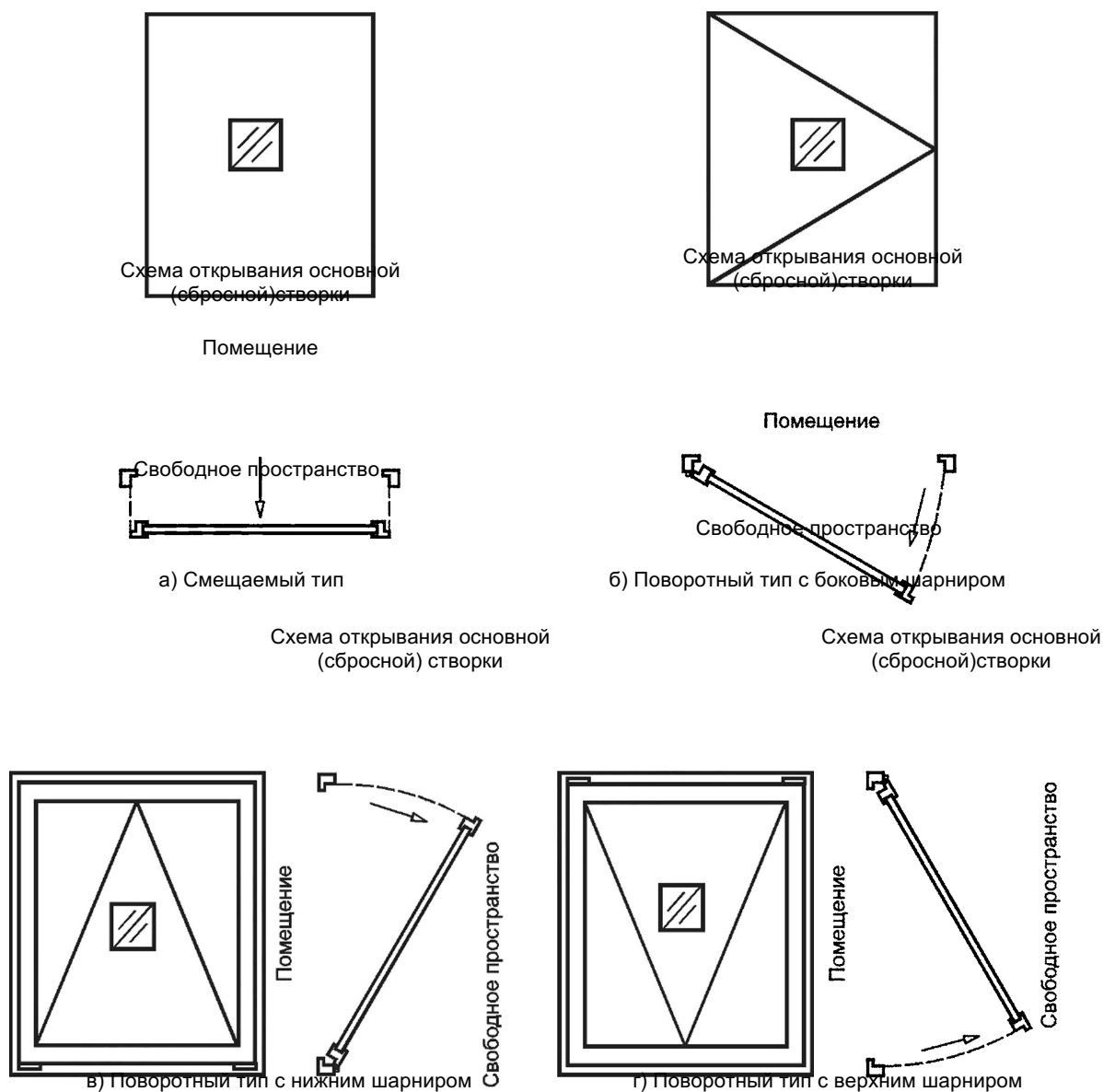
Рисунок 1 — Принципиальные схемы устройства ЛСКО
